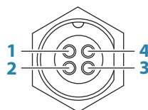
Enhetskontakt (hann)
