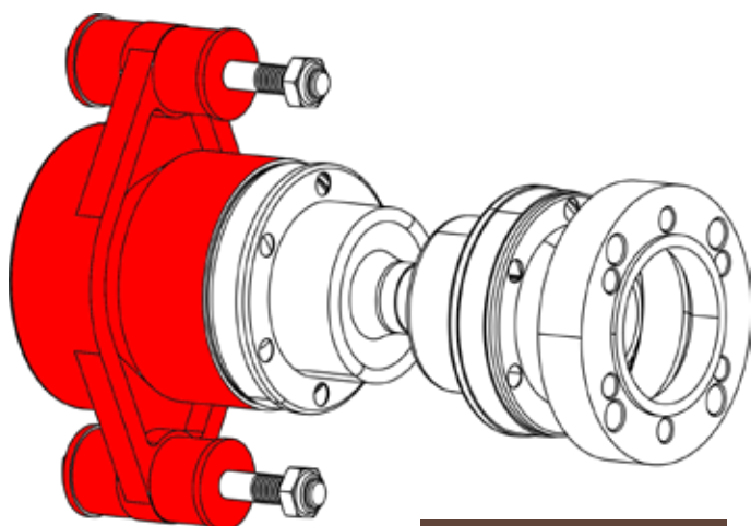
TRYKKLAGER
