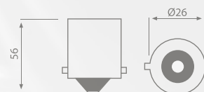
BA 15s
