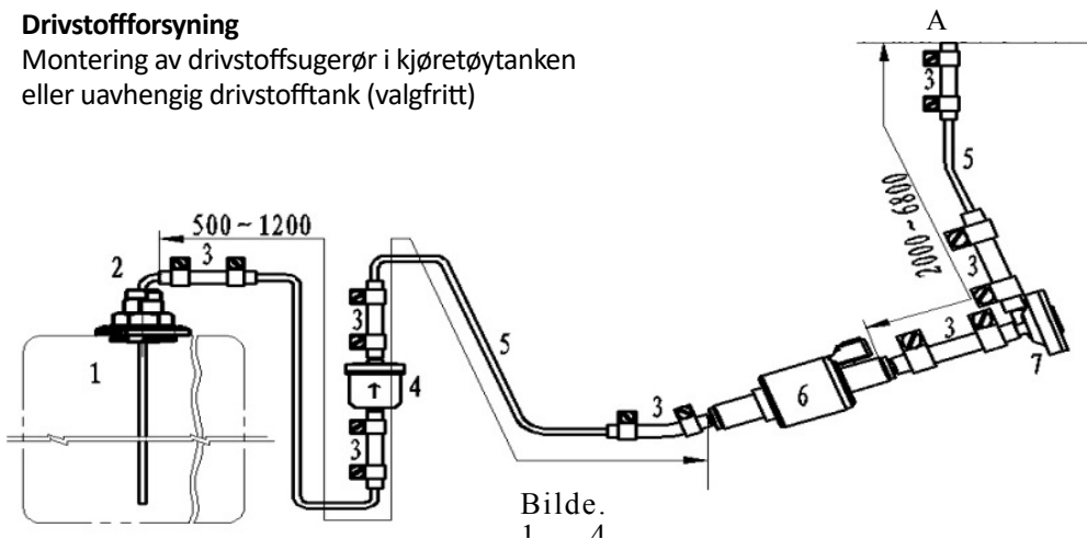
1-Drivstofftank 2- DrivstoffEkstraktor 3-Drivstoffr kontakt 4-Drivstoffrør 5-Filter6-Drivstoffpumpe (andre)7-Demper A- Fuel røroverflate
