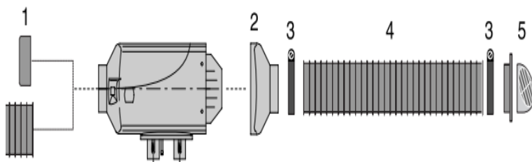
1-Sikkerhetsgitter 2 Hus-Utstrømningshette 3- slangeklemme - 4-Fleksibel slang 5- Roterendeutstrømning
