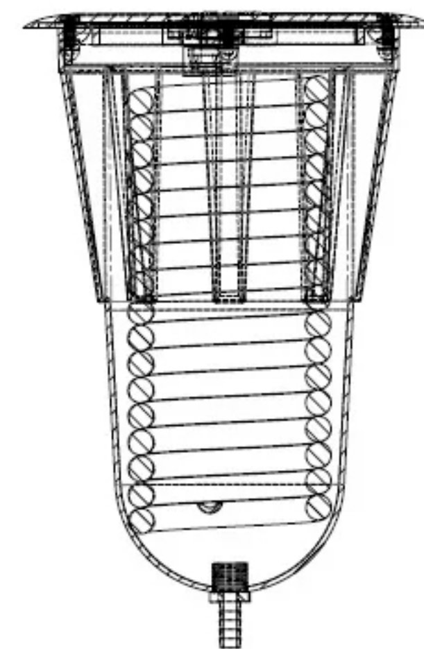
SECTION B-B SCALE 1 : 2
